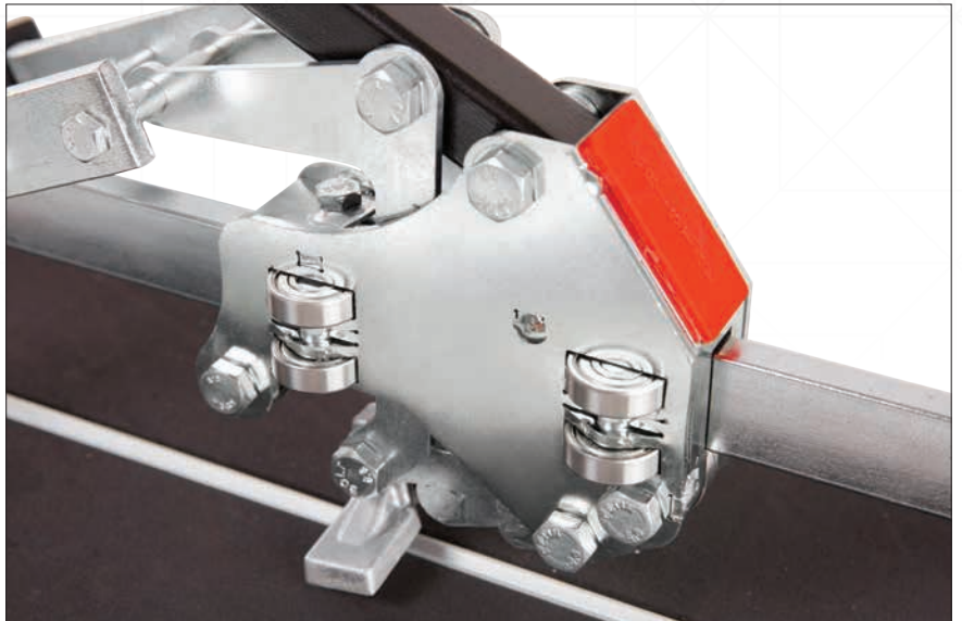
Kol mekanizması 11 adet kapalı bilyalı rulmandan oluşur.
