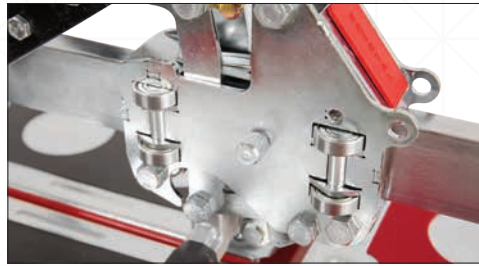
Kol mekanizması 13 adet kapalı, bilyalı rulmandan oluşur.
