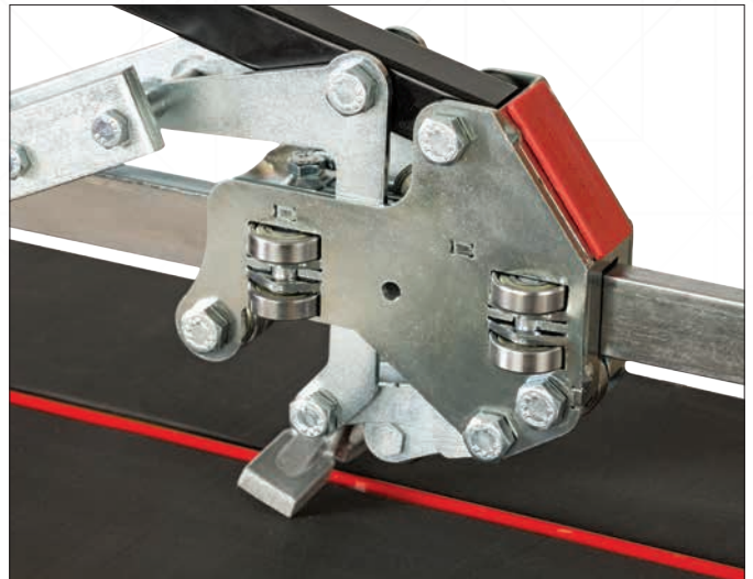
Kol mekanizması 11 adet kapalı bilyalı rulmandan oluşur.
